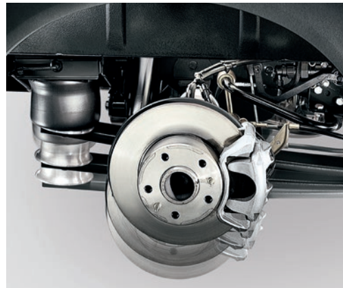
ЗАДНЯЯ ПНЕВМАТИЧЕСКАЯ ПОДВЕСКА
